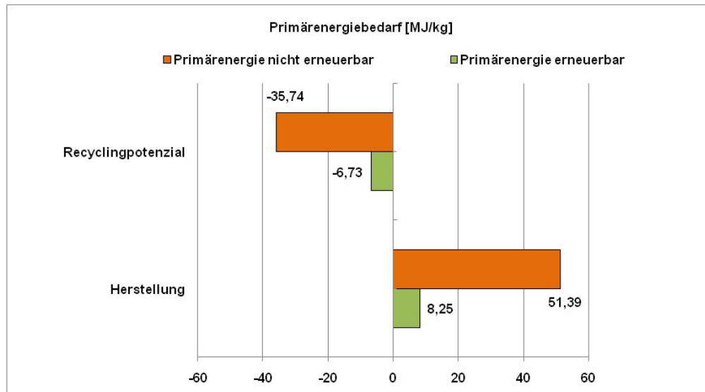
Abbildung 2: Bilanz für Primärenergieverbrauch je kg QUARTZ-ZINC® / ANTHRA-ZINC®
